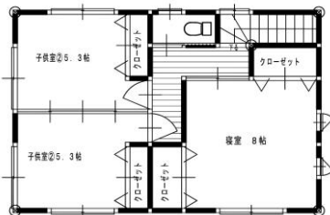
2階平面図
